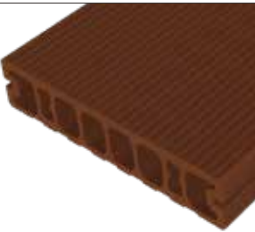
デッキ材断面図
