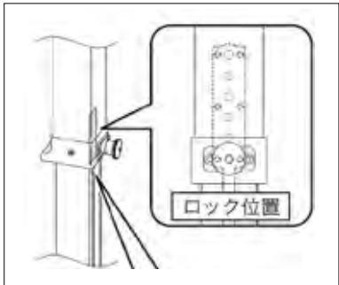
設置場所面の水勾配に対応した、 H調整 6 段階
