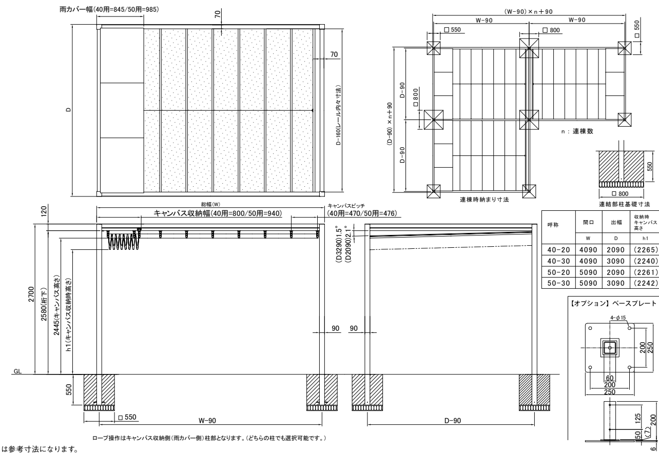
自立型 リパーロ 据え置き式 基本寸法図
