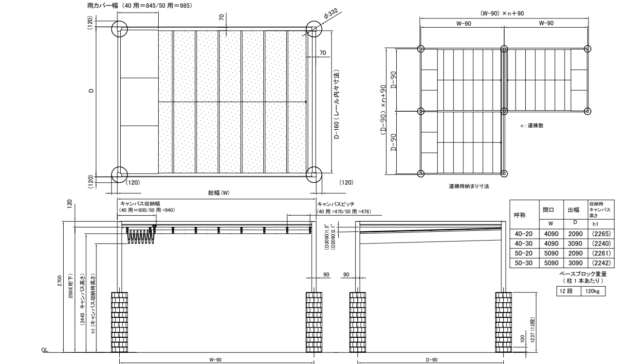
自立型 リパーロ 据え置き式 基本寸法図
