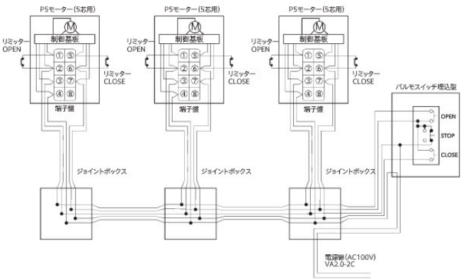
配線図
