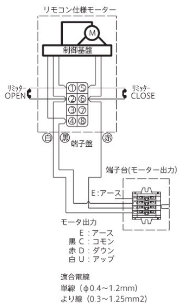
配線系統図
