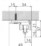
天井シングルブラケット付 (ブラケット幅=19mm)
