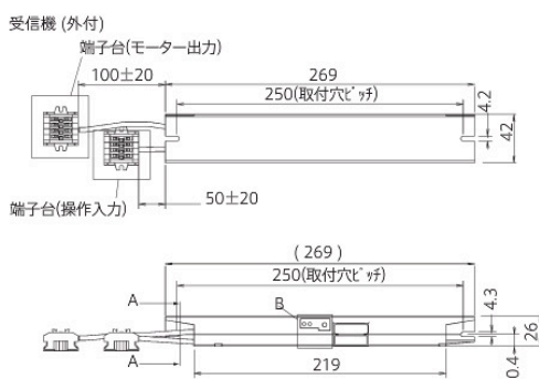
FMリモコン送受信機/寸法図
