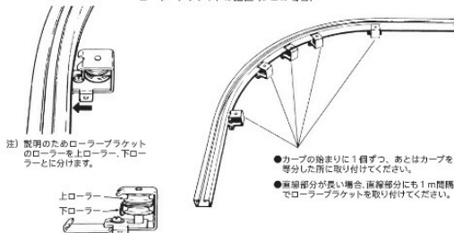
ローラーブラケットの配置 (5コの場合)
