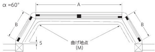
台形カーブレール (ダブル付)
