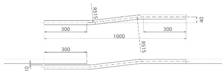
交叉レール
