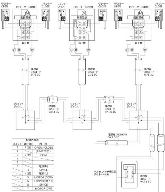
配線系統図
