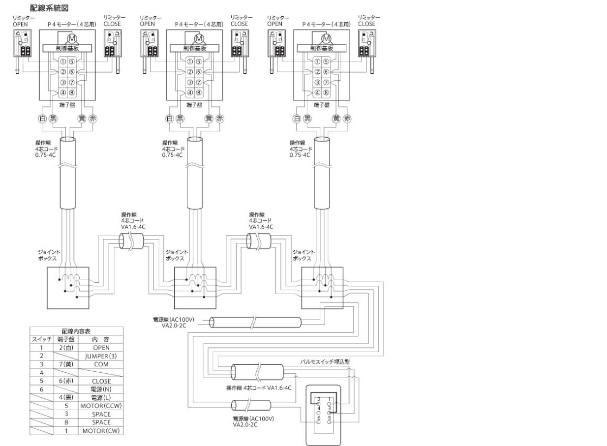
ニューII型・マキシマ 配線図
