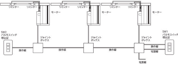
P4 モーター (4 芯) 一斉両面操作パルモスイッチ (増込)
