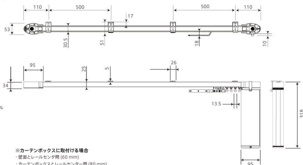
グリディア 取付寸法図 (単位: mm)
