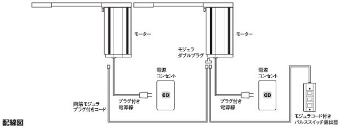
配線図
