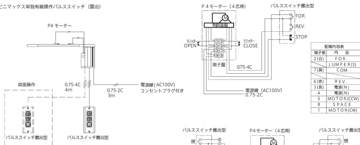
ビニマックス単独有線操作パルススイッチ（露出）
