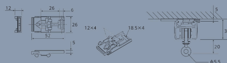
ブラケット寸法図
