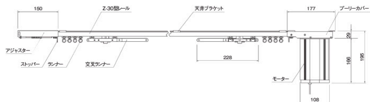
ミディアム取付寸法図 (Z-30)
