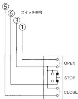
配線図
