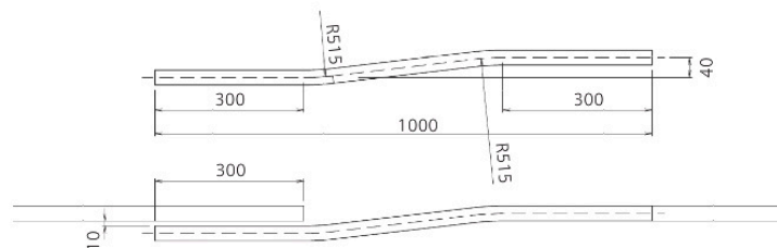
交叉レール
