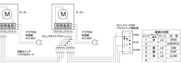
配線図
