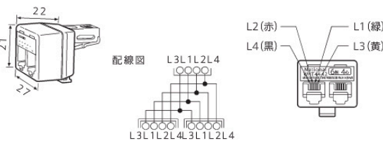
モジュラ関係部品寸法図
