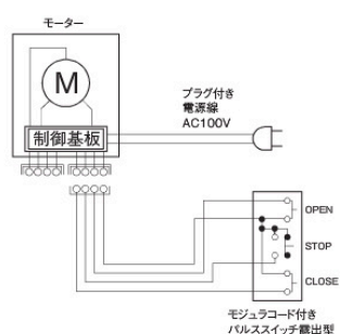
ミディアム配線図
