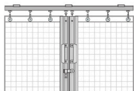
両開き間仕切フレーム2本タイプ
