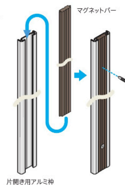
片開き納まり図
