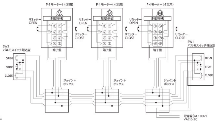
配線図
