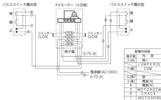
配線系統図
