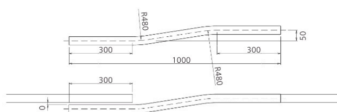
交叉レール
