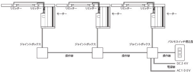
P6モーター (DC24V) 一斉操作/バブルモススイッチ (埋込)
