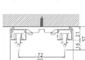
天井ダブルブラケット付 (ブラケット幅=18mm)
