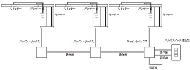
配線図
