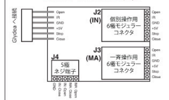
● DCTスプリッタのピン配置
