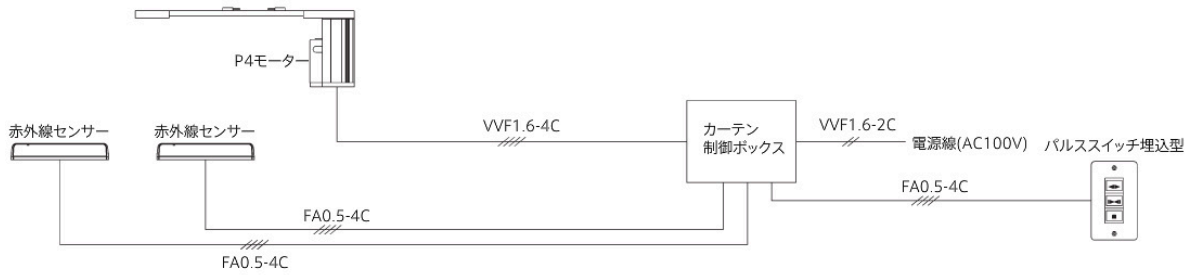
P4 モーター配線図
