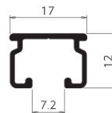
レール断面図 (mm)
