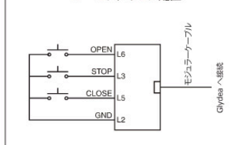
ローゼットのピン配置
