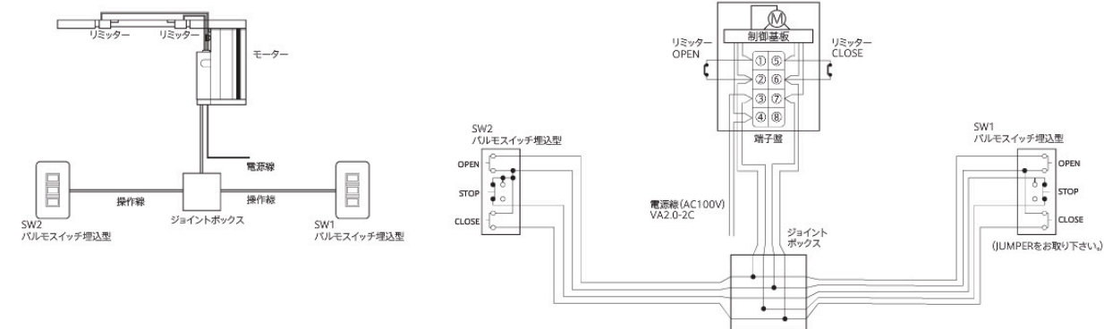
P4 モーター (4 芯AC付) 両面操作パルススイッチ (埋込)
