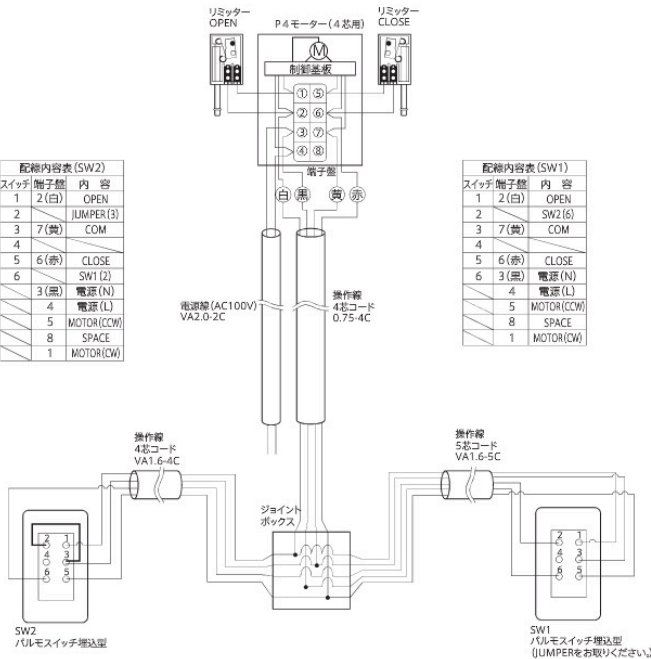
配線系統図
