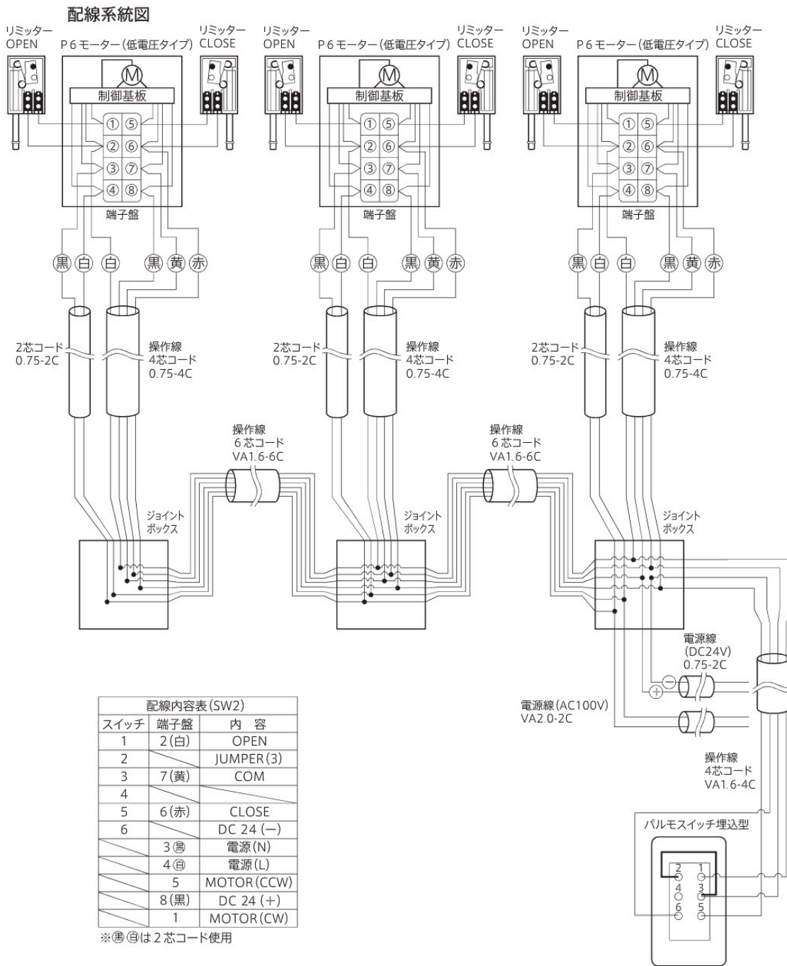
ニューII型配線図
