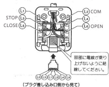
結線図
