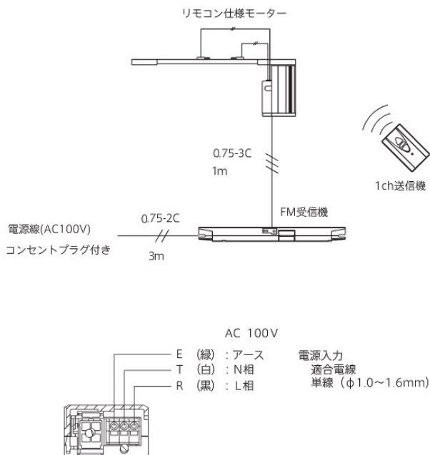
ビニマックス無線操作配線図
