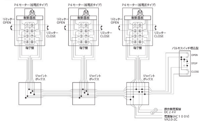
配線図
