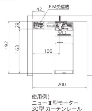
カーテンボックス納まり図 (天井ブラケット付)
