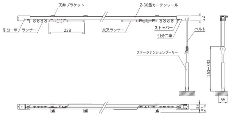
30 型紐引きカーテンレール寸法図
