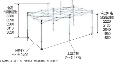
フレーム
