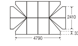
天幕(平面図)
