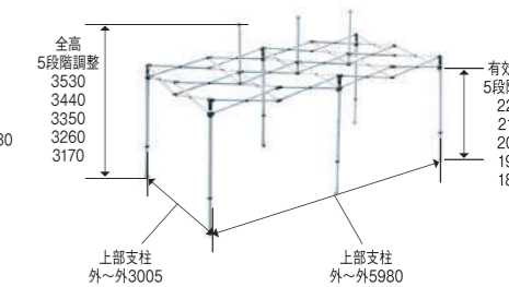
フレーム
