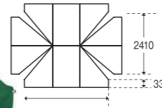
天幕(平面図)
