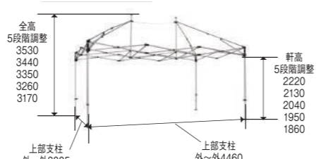
フレーム
