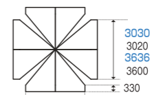
天幕(平面図)
