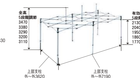
フレーム
