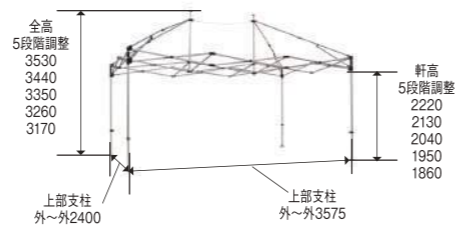
フレーム
