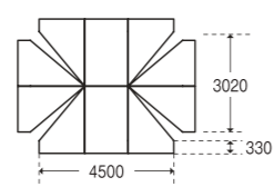
天幕(平面図)
