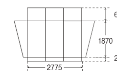
天幕(平面図)
