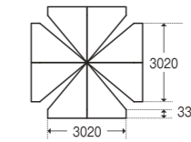
天幕(平面図)
