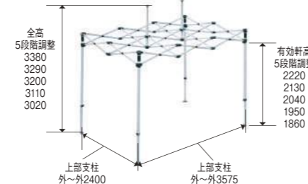
フレーム
