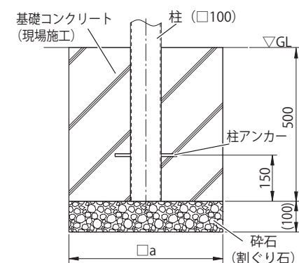
[2] 基礎の種類 ※ ( ) 寸法は目安寸法となります。
