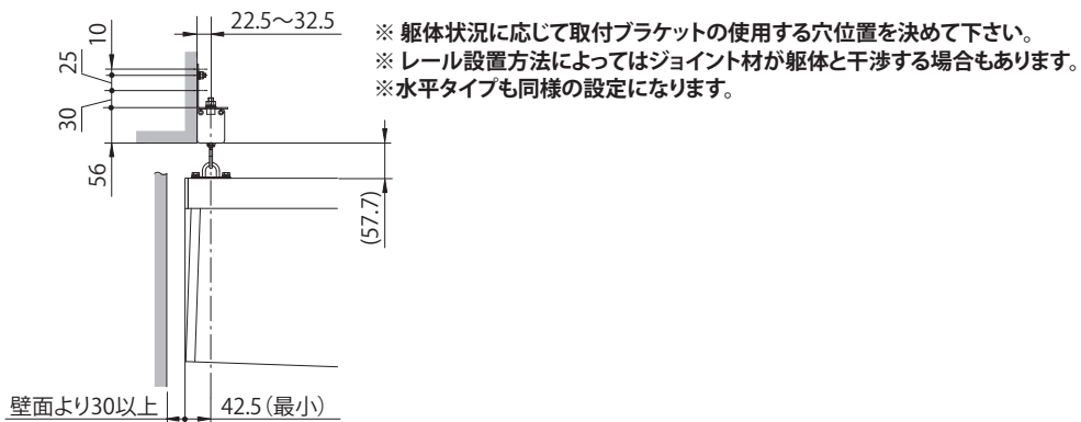
【取付例②】※（ ）寸法は目安寸法となります。 ※【キャンパスバーにジョイント材を使用時の注意】 規格別重量表を参照して下さい。
