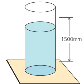
(図8) 耐水試験の原理 上記試験で水準装置が1500mm高の時の水圧は、生地の上に円筒を固定して水を注いでいき、水位が1500mmになった時に生地にかかる水位とひとしい。
